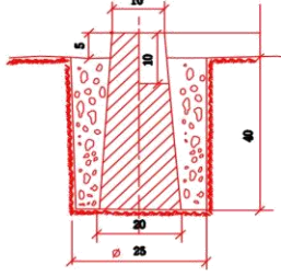
YUMUŞAK ZEMİNDE PARSEL KÖŞESİ TESİSİ
