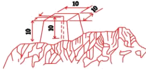
BLOK KAYALIK ZEMİNDE PARSEL KÖŞESİ TESİSİ
