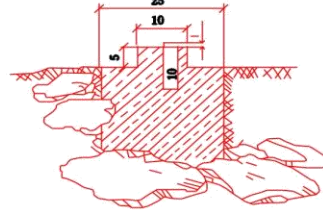
GEVŞEK KAYALIK ZEMİNDE PARSEL KÖŞESİ TESİSİ
