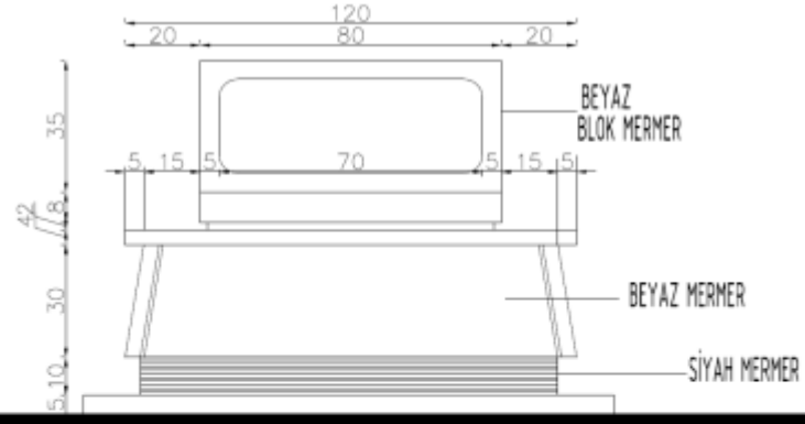
TİP MEZAR ÖN GÖRÜNÜŞ
