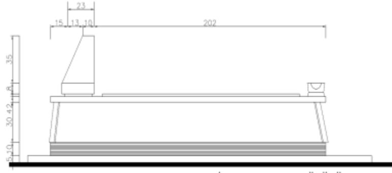
TIP MEZAR YAN GÖRÜNÜŞ
