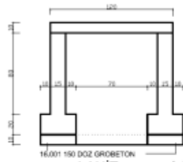
LAHİT A - A KESİTİ
