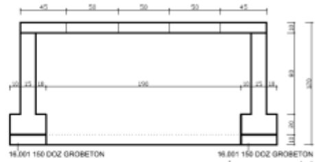
LAHİT B - B KESİTİ
