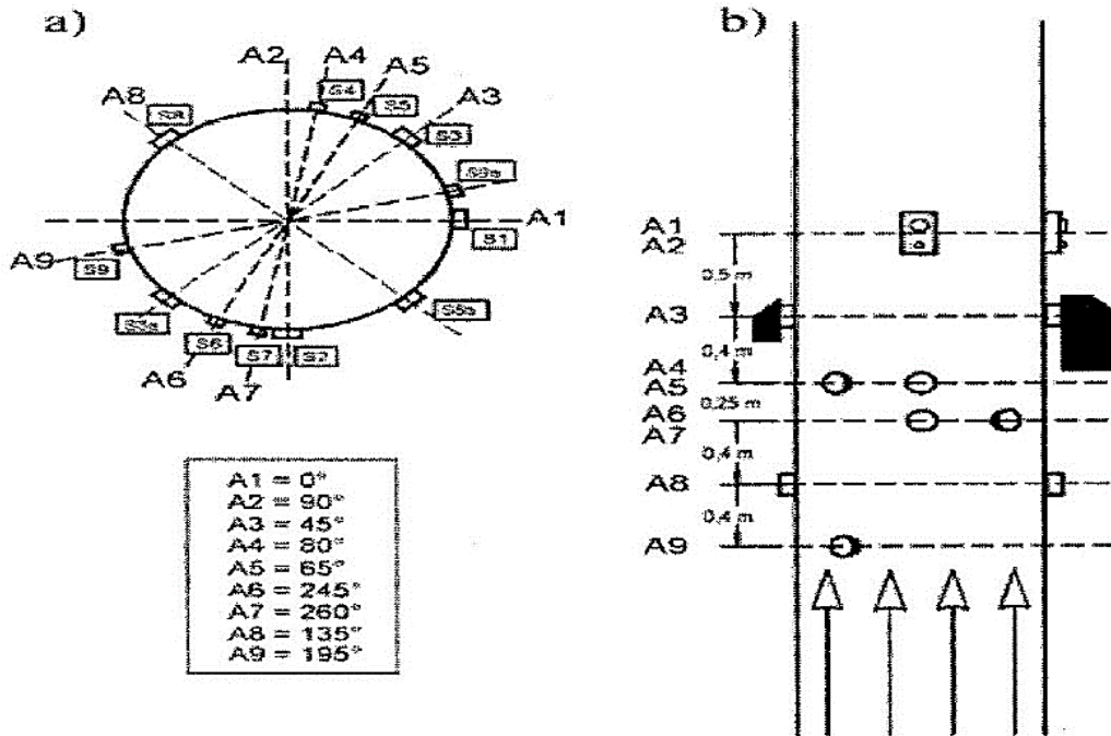
Şekil 3: Numune alma noktaları için örnek yerleşim planı
