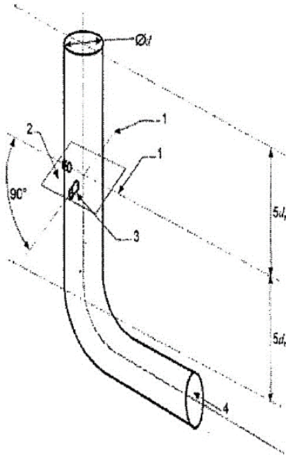
Şekil 1: Numune alma hattı ve düzlemi
